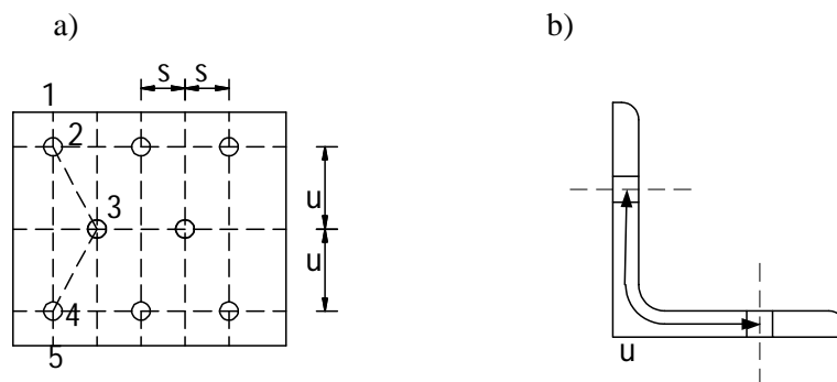
Hình 1 – Cách xác định diện tích thực
