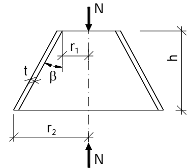
Hình 17 – Sơ đồ vỏ nón tròn xoay chịu lực nén dọc
