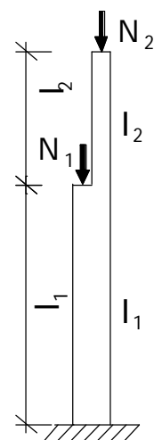
Hình D.1 – Sơ đồ cột một
